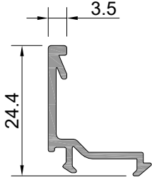
Profil No: W-511-a ⚠ Ağırlık : 193 gr/m ⚠ İşaretili profil için satış temsilcilerinizden bilgi alınız.
