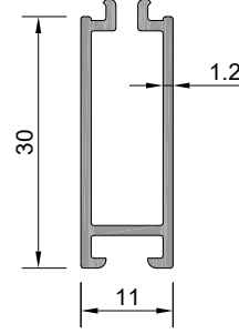
Profil No : KC0352 ⚠ Ağırlık : 270 gr/m ⚠ İşaretli profil için satış ekibinden bilgi alınız.
