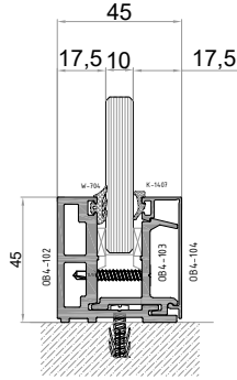
8 - DETAY
