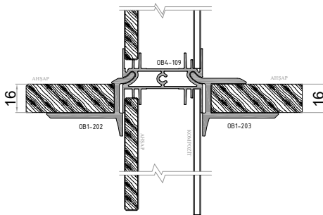
7 - DETAY
