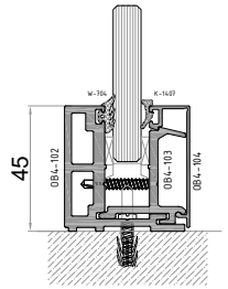
11 - DETAY
