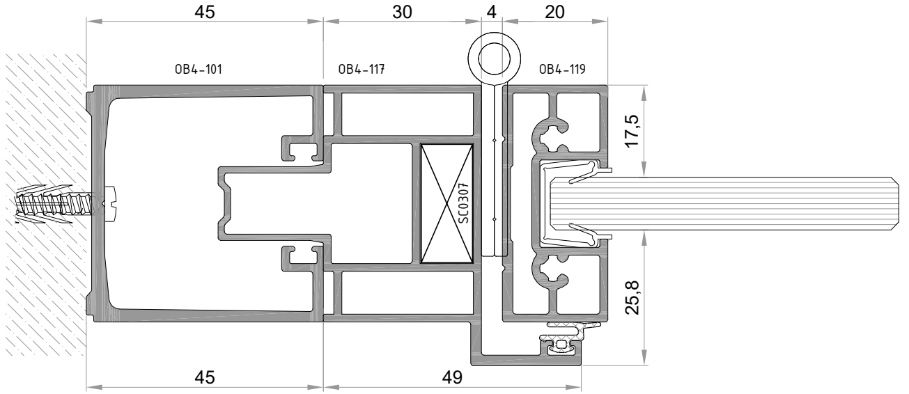
DETAY-3
