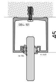
10 - DETAY
