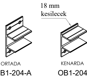
Profil No : OB1-204 Ağırlık : 963 gr/m
