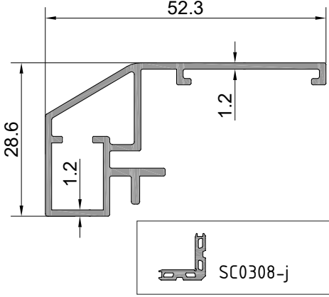
Profil No : OB1-110 Ağırlık : 487 gr/m
