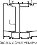
SÜPÜRGELİK GÖVDE VE KAPAK İMALAT ÖLÇÜLERİ
