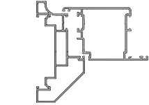
KAPI KASA İMALAT ÖLÇÜSÜ
