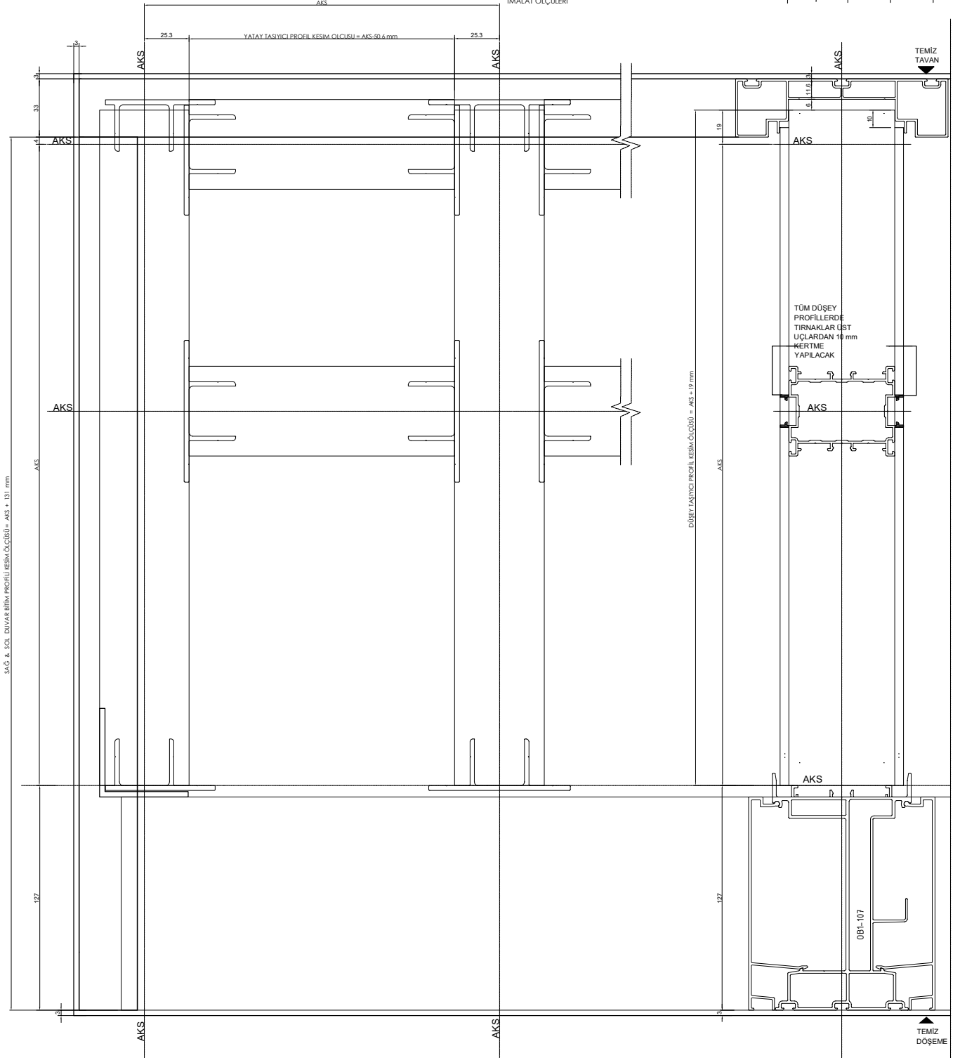
YATAY VE DÜŞEY TAŞIYICI PROFİL İMALAT ÖLÇÜLERİ
