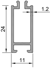
Profil No : KC0347 Ağırlık : 233 gr/m
