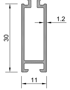
Profil No : KC0352 ⚠ Ağırlık : 270 gr/m ⚠ İşaretili profil için satış ekibinden bilgi alınız.
