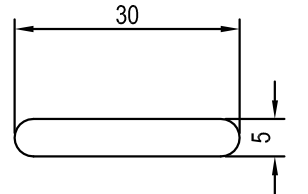
TAHLİYE DELİĞİNİN ÖLÇÜLERİ DRAINAGE HOLE DIMENSIONS
